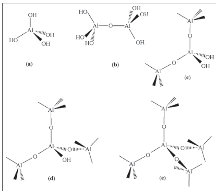
Figura 5: Esquema das estruturas de algumas espécies de alumínio: (a) [\text{Al}(\text{OH})_4]^- ; (b) [\text{Al}_2\text{O}(\text{OH})_6]^{2-} ; (c) [\text{Al}(\text{OH})_2(\text{OAl})_2]_x^- ; (d) [\text{Al}(\text{OH})(\text{OAl})_3]^{3-} ; (e) [\text{AlO}_3]^- . Adaptado da ref. 23
